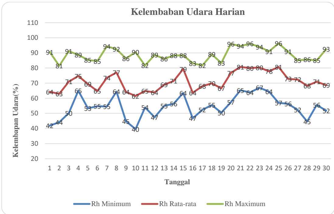
Gambar 13. Grafik Kelembaban Udara Harian
