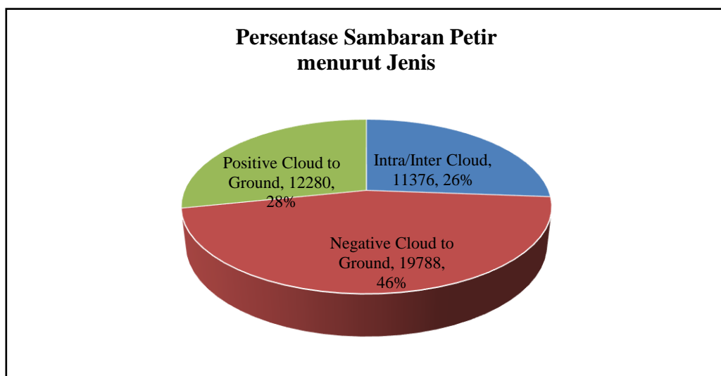
Gambar 5. Total Sambaran Menurut Jenis Muatan
