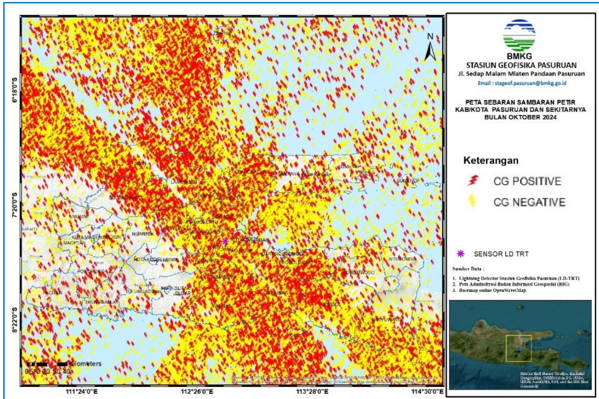
Gambar 9. Peta Intensitas Sambaran Petir di Wilayah Kabupaten Pasuruan dan Sekitarnya Bulan Oktober 2024.
