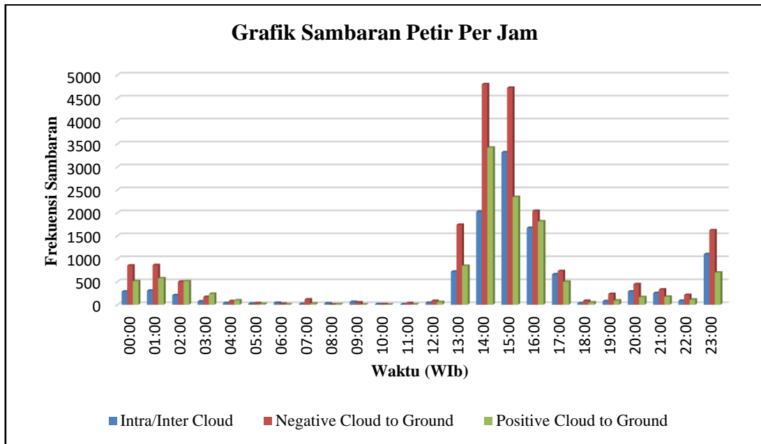
Gambar 8. Grafik Jumlah Sambaran Petir Per Jam
