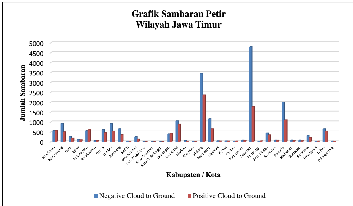
Gambar 7. Grafik Jumlah Sambaran Petir Wilayah Jawa Timur
