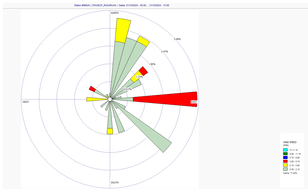
Gambar 14. Grafik Wind Rose
